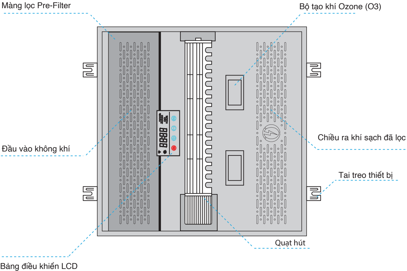
Mô phỏng cấu tạo thiết bị OzoneTech OTK-CS10GH
